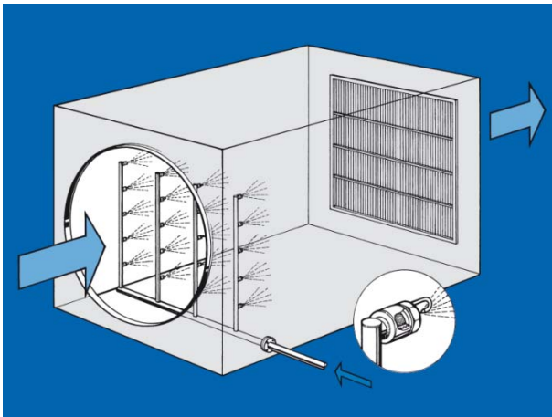
Hochdruckbefeuchter Typ HPH
